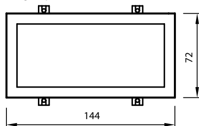
Disegno quotato A
